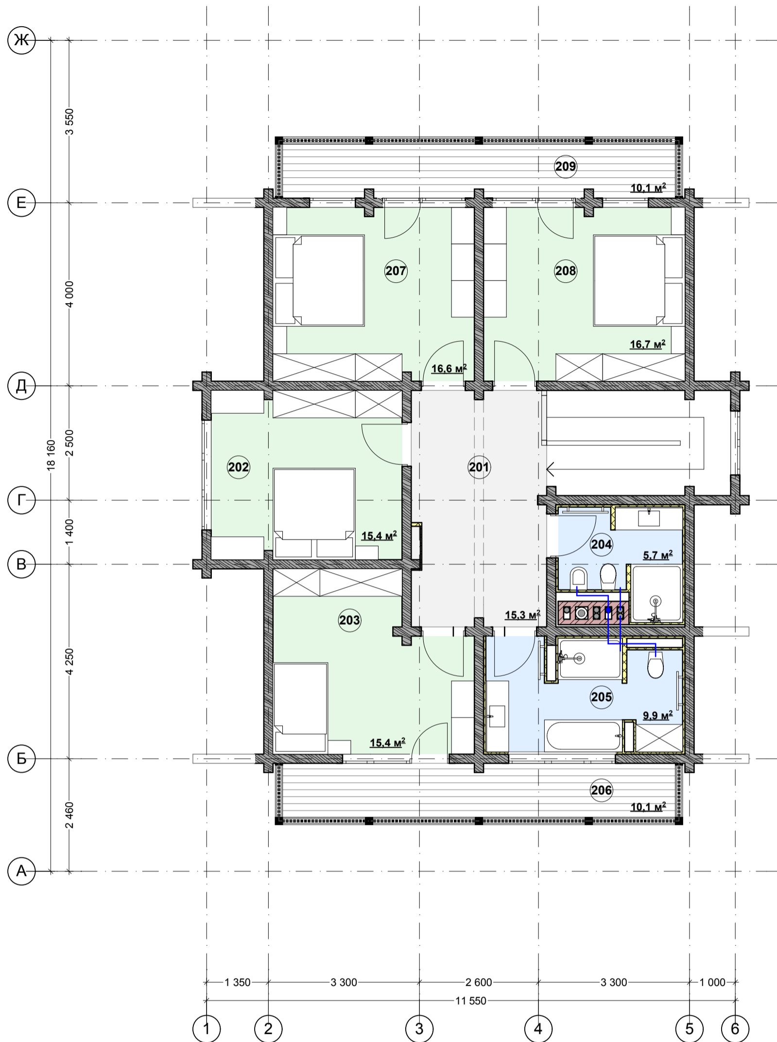
Экспликация помещений 2-го этажа
